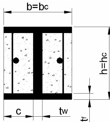
Figura 7.6.1 - Rapporti dimensionali
